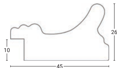
Profil lišty 1:1
