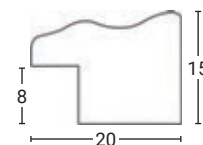
Profil lišty 1:1
