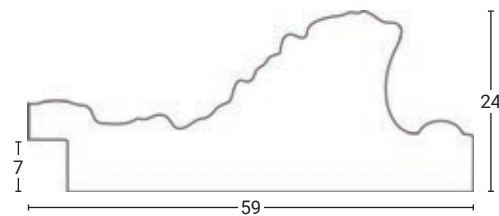
Profil lišty 1:1
