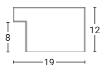
Profil lišty 1:1
