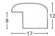
Profil lišty 1:1
