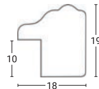
Profil lišty 1:1
