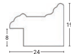
Profil lišty 1:1
