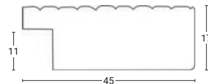
Profil lišty 1:1
